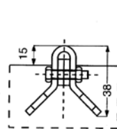
SOLUZIONE CON BINARIO SPORGENTE DAL PAVIMENTO
