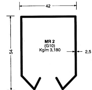
MR 2 "B" (MEDIA) Tipo per carrelli piccoli
